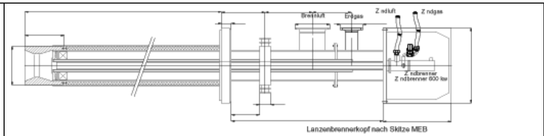
Temperbrenner 0,8 MW
