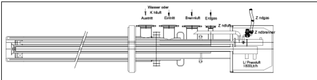
Öl-Gas-Lanzenbrenner mit Wasser oder Luftkühlung oder Feuerfestisolierung. Leistung bis 60 MW. (Andere Leistungen auf Anfrage)
